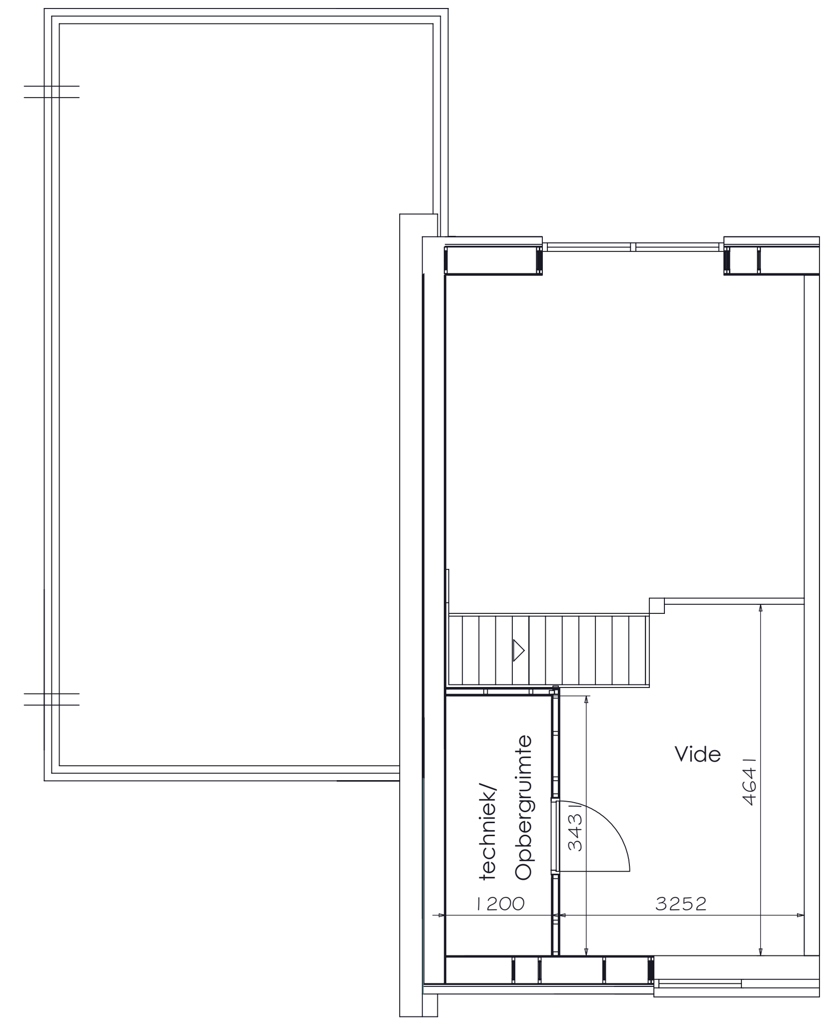
Eerste etage
